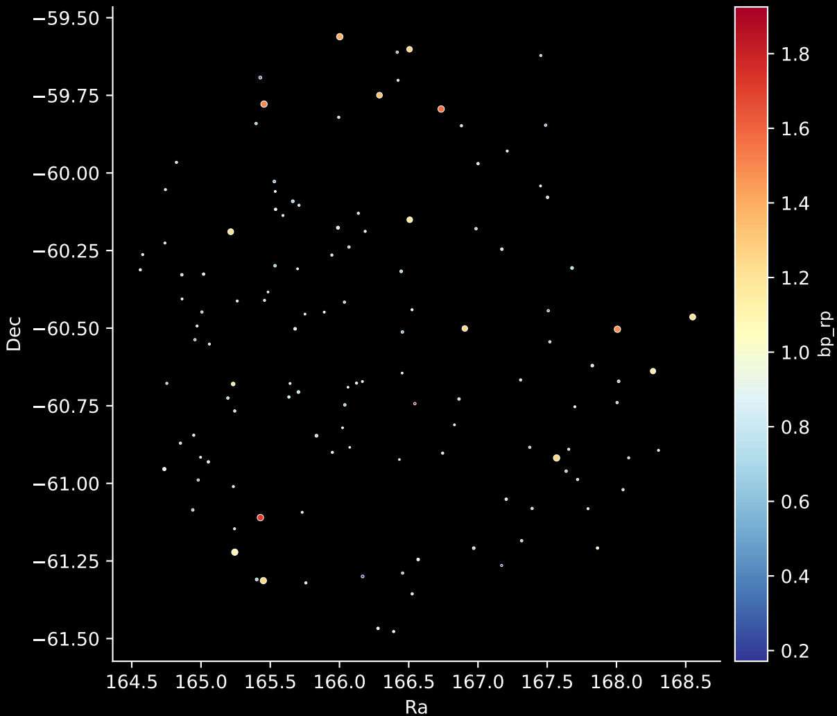
GALAH DR4 Field: [7212] Stars: 125
