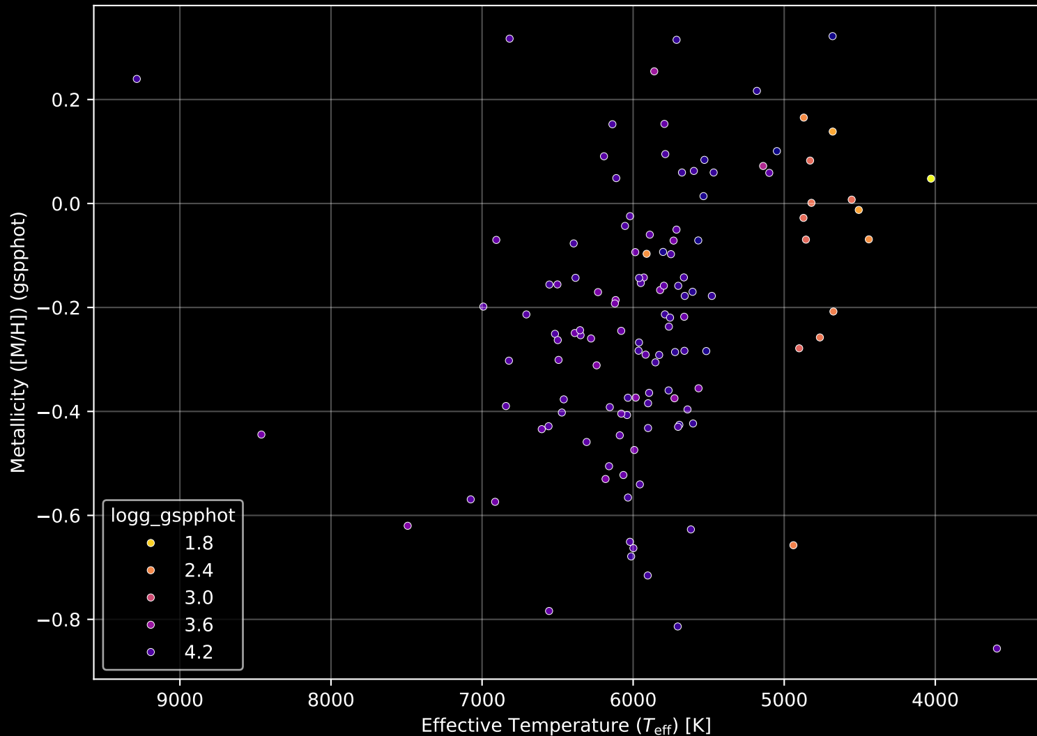
GALAH DR4 Field: [7212] Stellar Population Parameters (n= 125)
